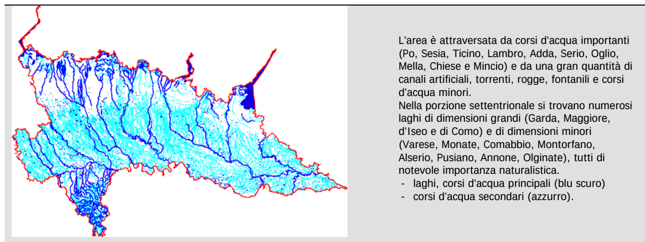
Figura 21 Reticolo idrografico
