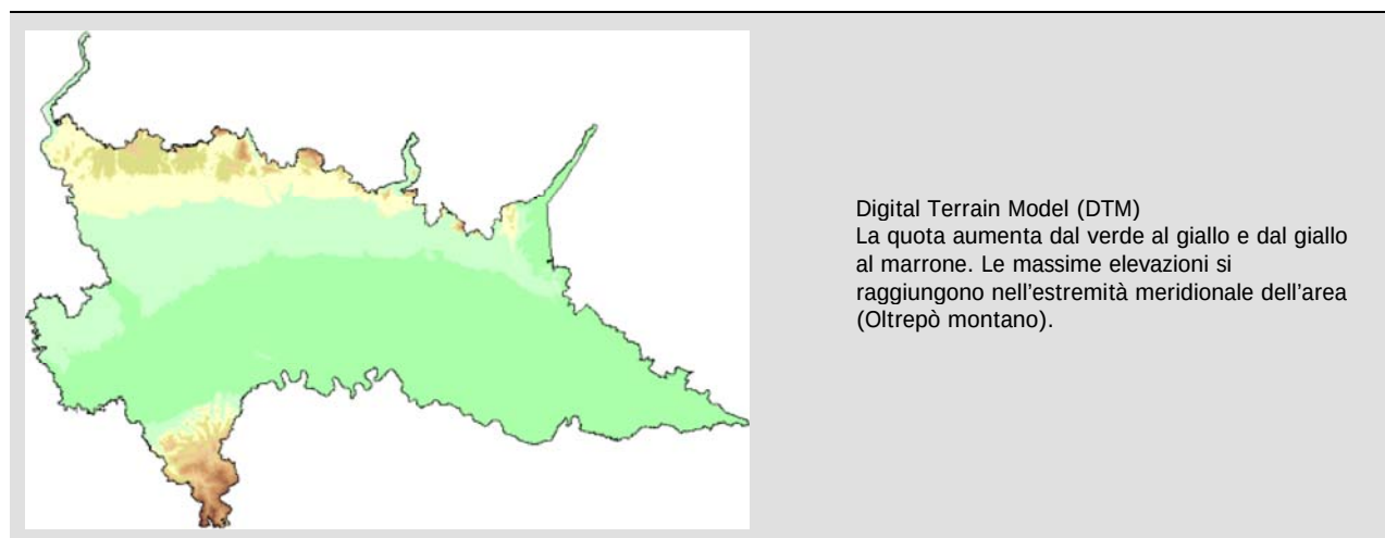
Figura 20 Quote altimetriche
