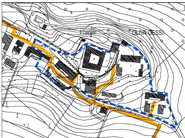
Figura 11. La rete del gas: Oliva Gessi
