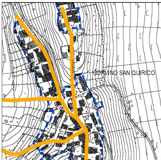
Figura 1. La rete fognaria: Corvino San Quirico
