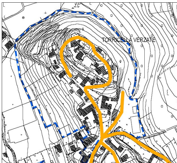
Figura 4. La rete fognaria: Torricella Verzate
