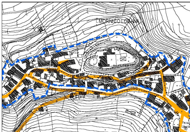
Figura 10. La rete del gas: Mornico Losana
