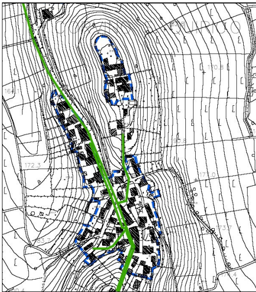
Figura 5. La rete dell'acquedotto: Corvino San Quirico
