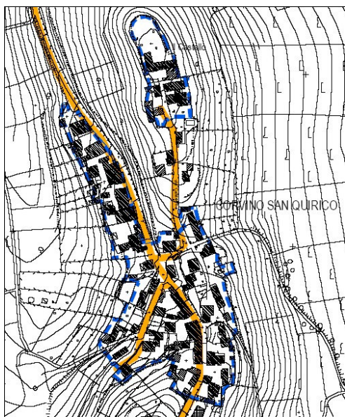
Figura 9. La rete del gas: Corvino San Quirico
