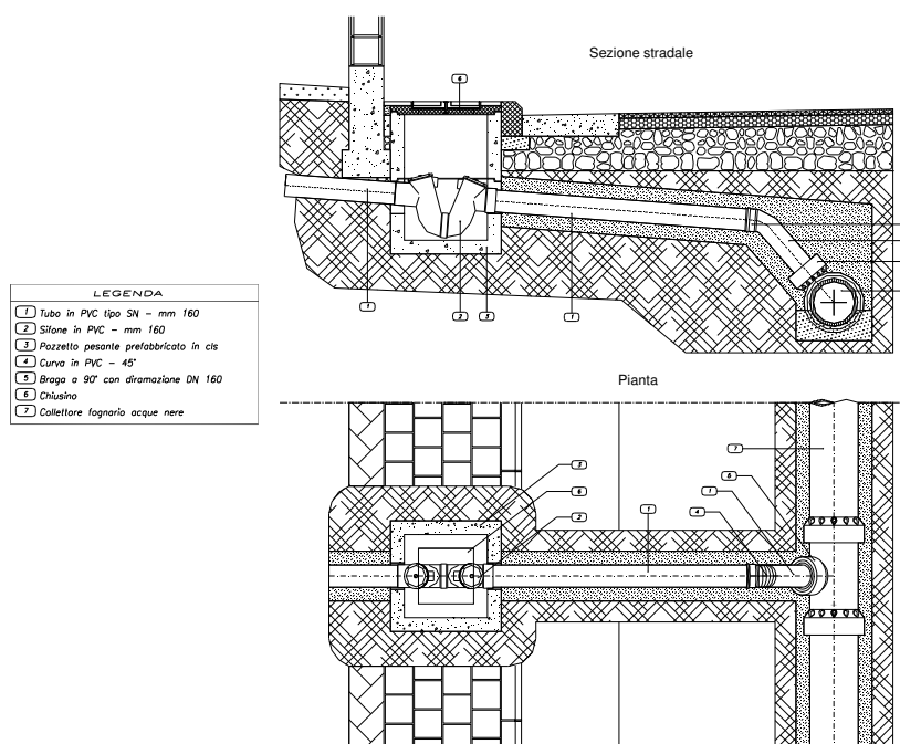
Figura 14. Allaccio tipo
