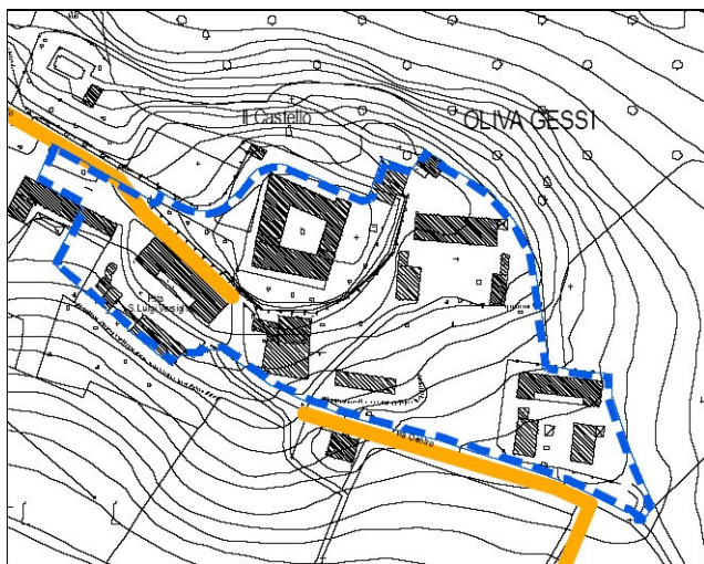
Figura 3. La rete fognaria: Oliva Gessi
