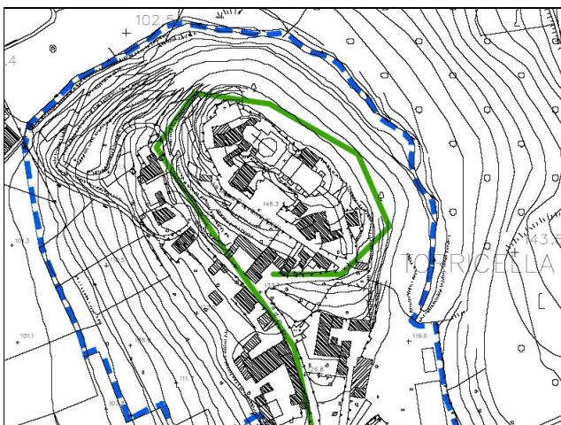
Figura 8. La rete dell'acquedotto: Torricella Verzate
